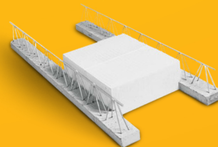
СБОРНО МОНОЛИТНОЕ ПЕРЕКРЫТИЕ
